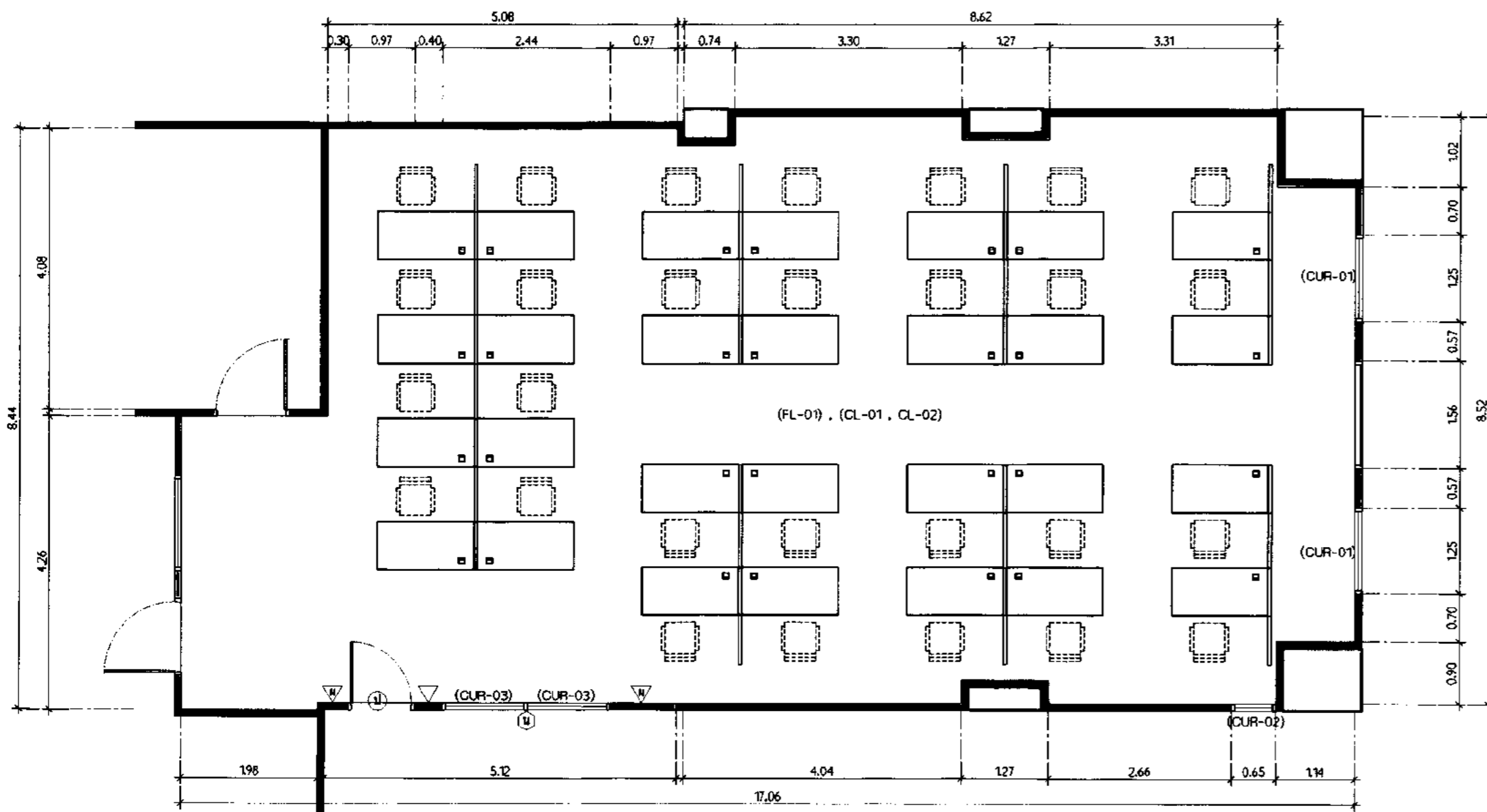
ผังครุภัณฑ์ห้องเก็บของขนาด 22 ตร.ม. และ ห้องเก็บของขนาด 84 ตร.ม. มาตราส่วน 1 : 75 (ปรับปรุงเป็นห้องทำงานที่ปรึกษา สมช. จำนวน 28 คน)
