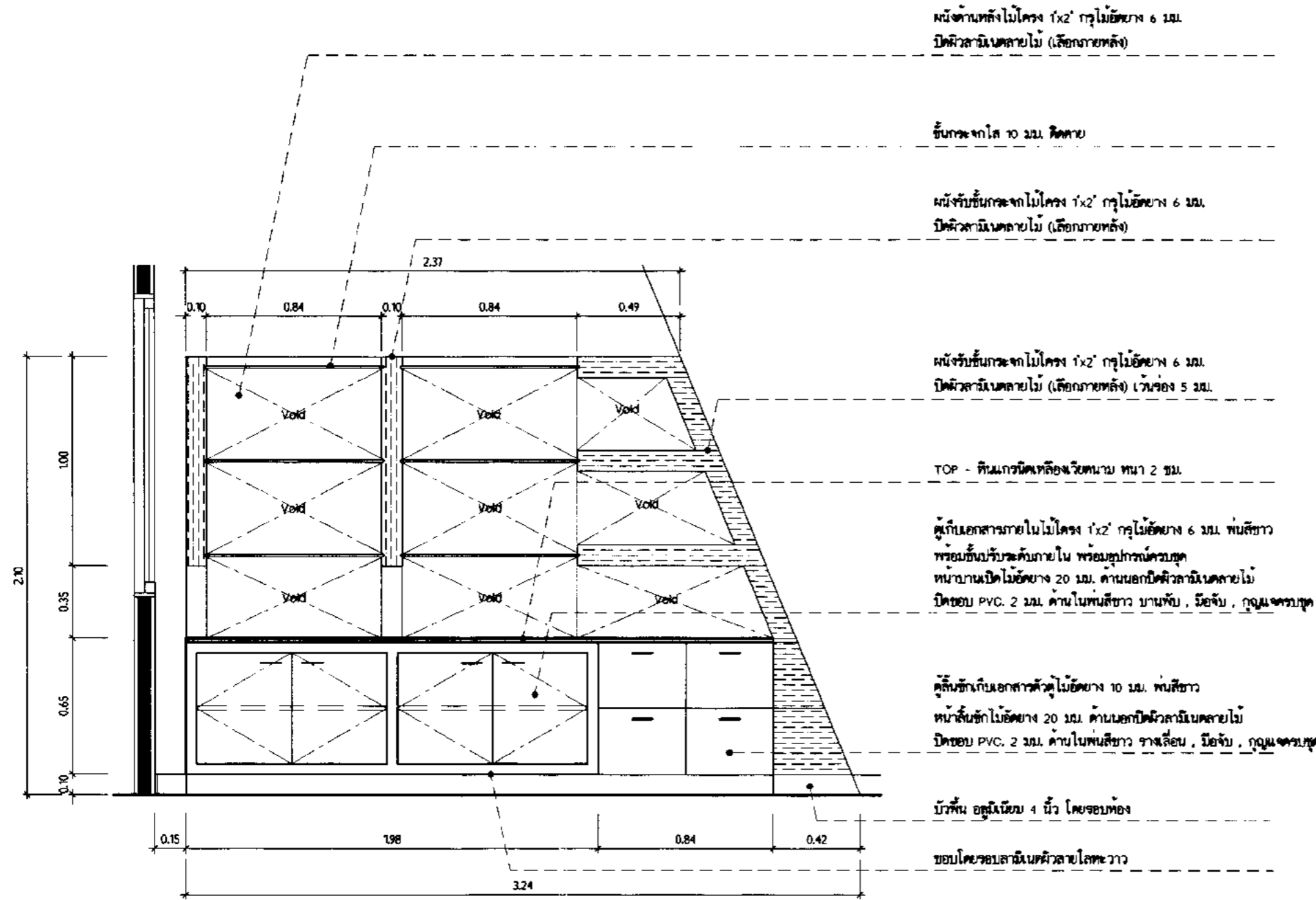
รูปติดตั้งหน้าครุภัณฑ์ (B-01) มาตราส่วน 1:25
