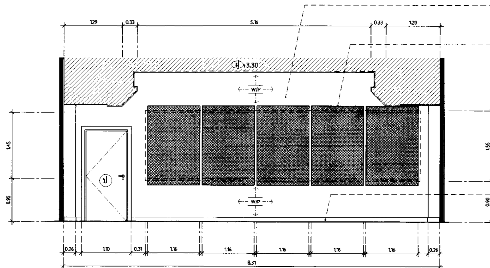
รูปตัดด้าน B มาตราส่วน 1:50
