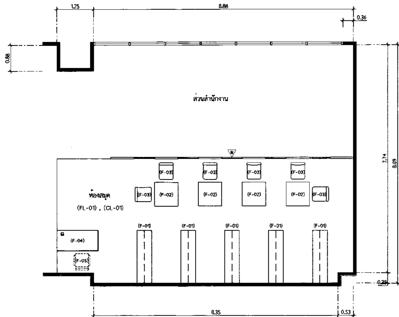
ผังกลุ่มพัฒนาองค์ความรู้ด้านความมั่นคง มาตราส่วน 1:50 (ปรับปรุงเป็นห้องสมุด)
