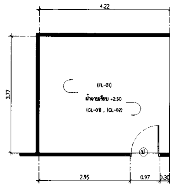
ผังพื้นที่ห้องนอน มาตราส่วน 1:50
