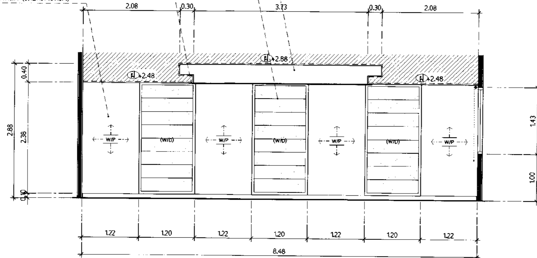
รูปตัดด้าน D มาตราส่วน 1:50
