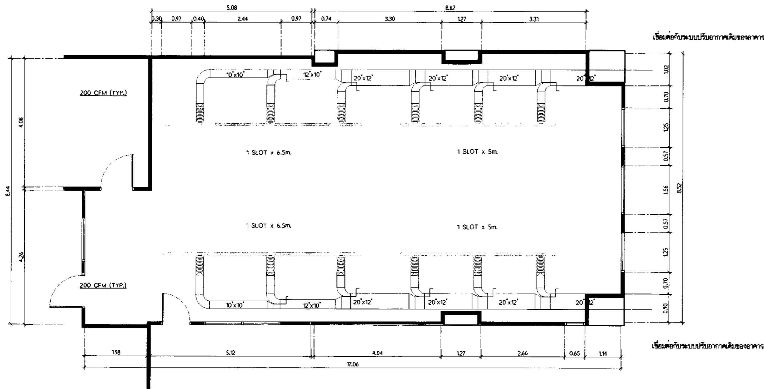
ผังงานระบบปรับอากาศห้องเก็บของขนาด 22 ตร.ม. และ ห้องเก็บของขนาด 84 ตร.ม. มาตรฐาน (ปรับปรุงเป็นห้องทำงานที่ปรึกษา สมช. จำนวน 28 คน) 1 : 75
