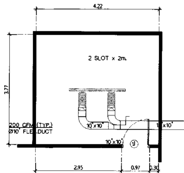
ผังต่อระบบปรับอากาศห้องนอน มาตราส่วน 1:50
