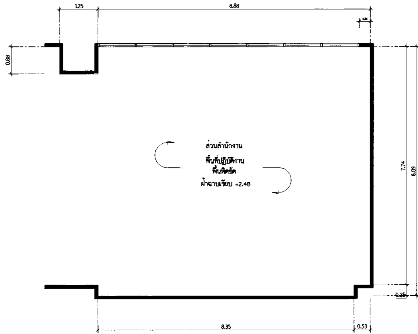
ผังกลุ่มพัฒนาองค์ความรู้ด้านความมั่นคง มาตราส่วน 1:50 (ผังสภาพปัจจุบัน)
