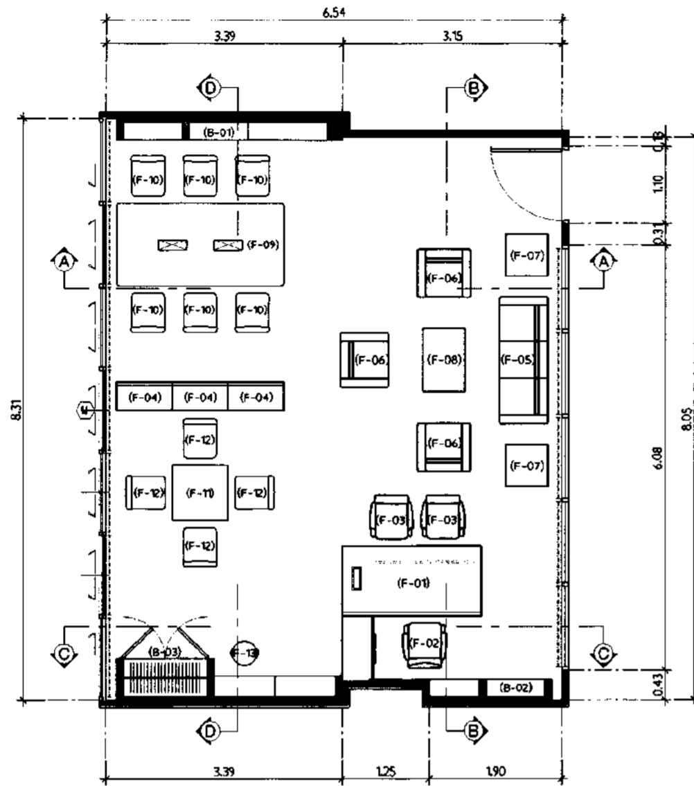
ผังครุภัณฑ์ห้องทำงานรองเลขาธิการ สมช. มาตรา ๗๗ 1:75
