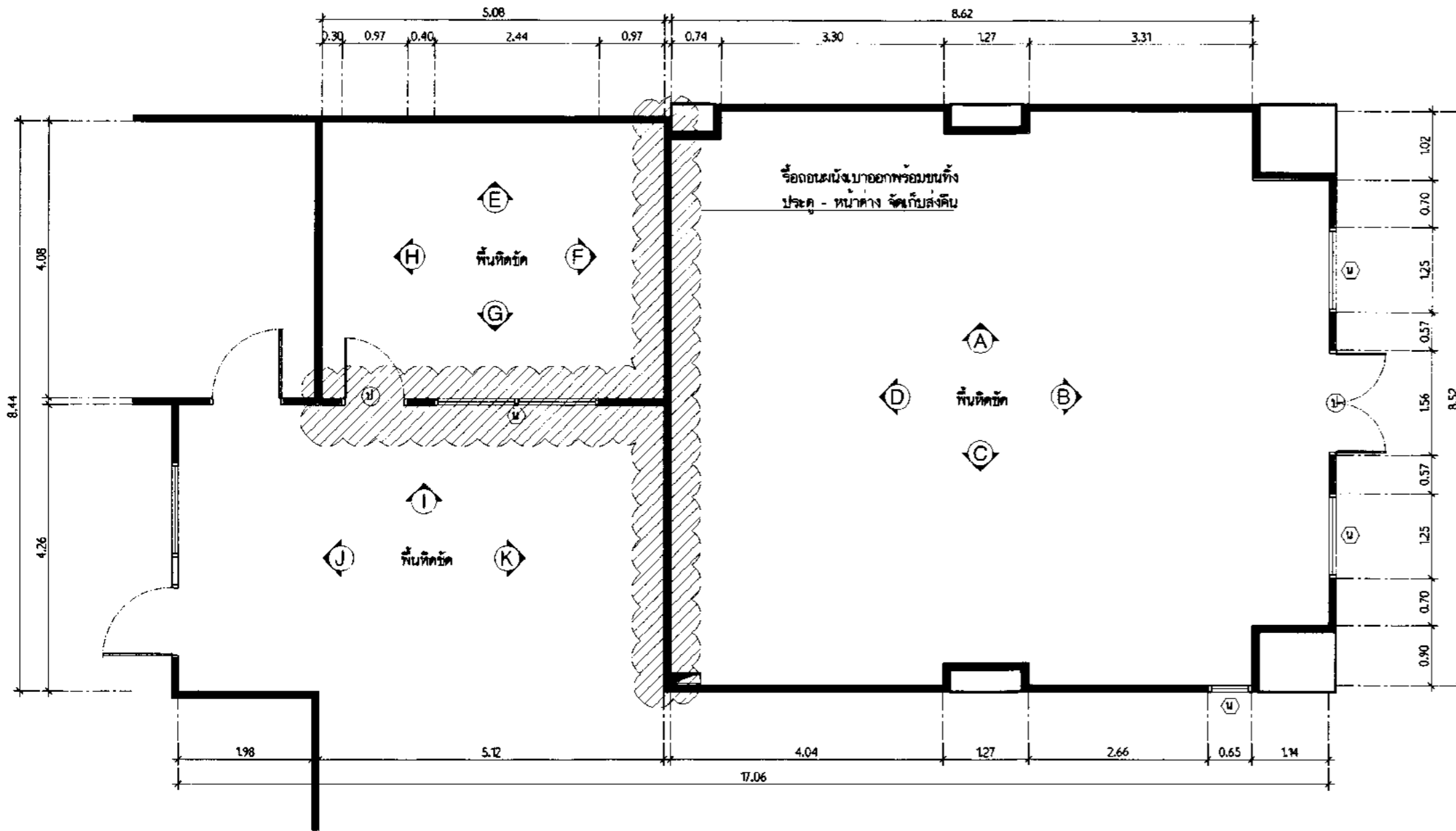
ผังพื้นที่ห้องเก็บของขนาด 22 ตร.ม. และ ห้องเก็บของขนาด 84 ตร.ม. (สภาพปัจจุบัน) มาตราส่วน 1 : 75 (ปรับปรุงเป็นห้องทำงานที่ปรึกษา สมช. จำนวน 28 คน)
