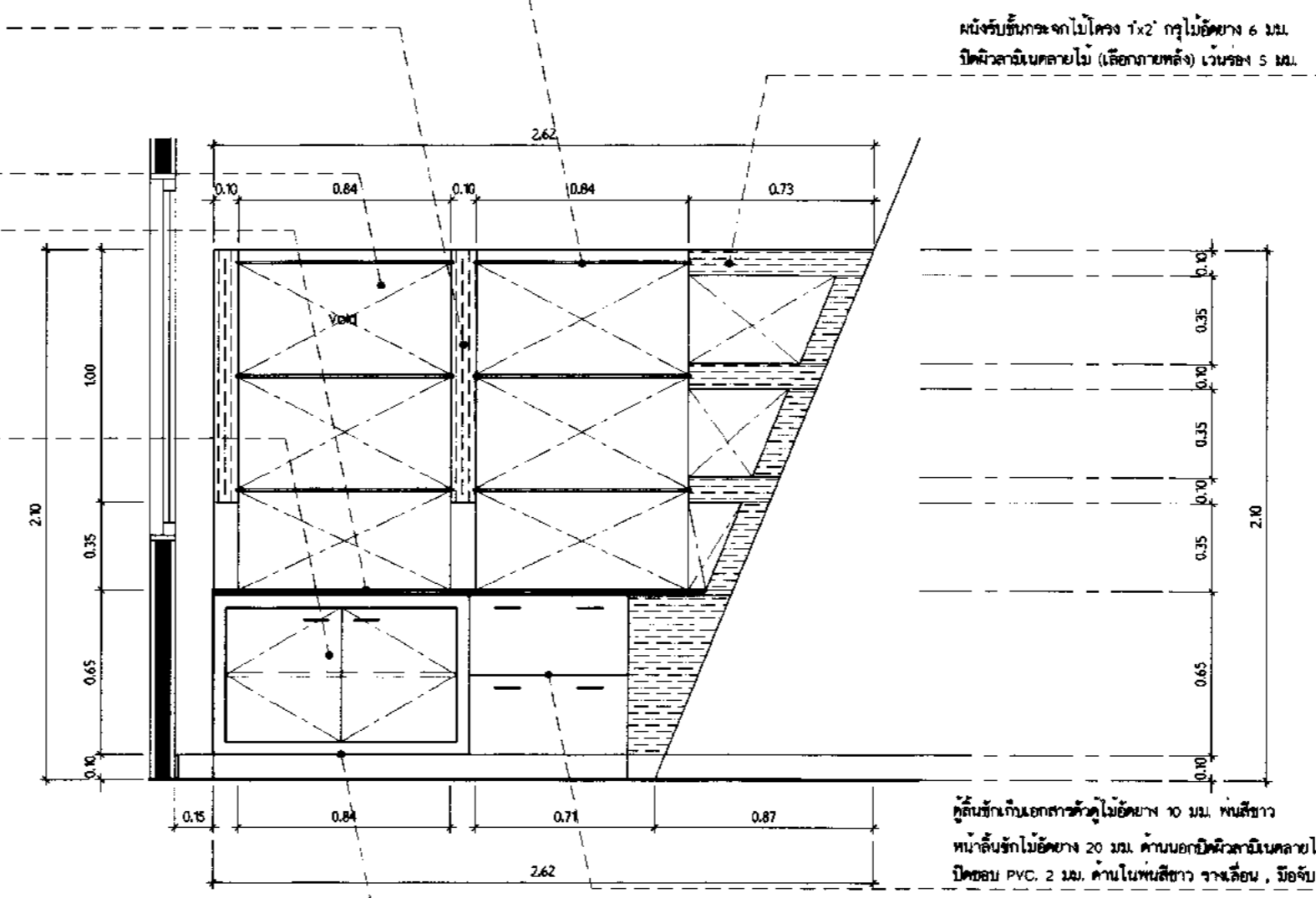
รูปตัดด้านหน้าครุภัณฑ์ (B-02) มาตรฐาน 1 : 25
