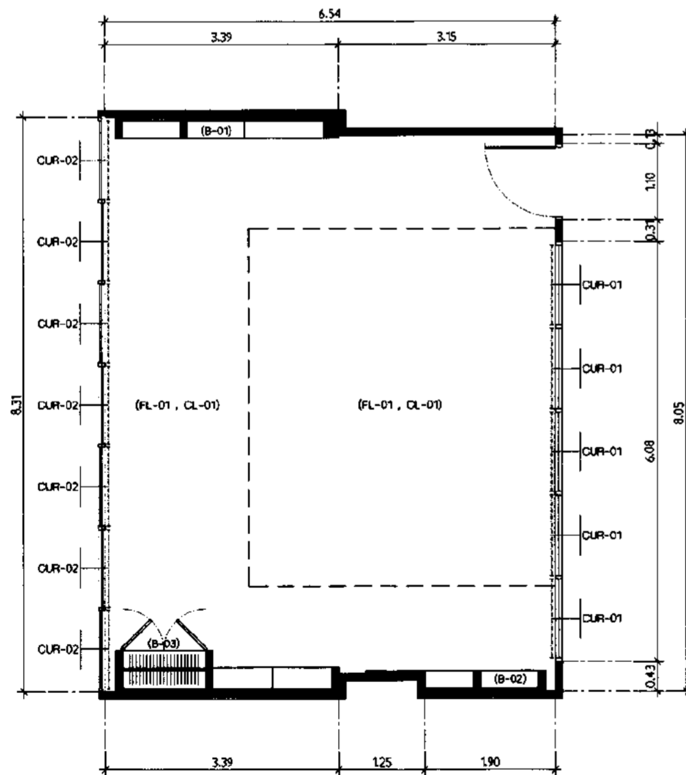
ผังครุภัณฑ์ห้อง สมช.มณ./สอ.กทอ. มาตรา ๗๗ 1:75
