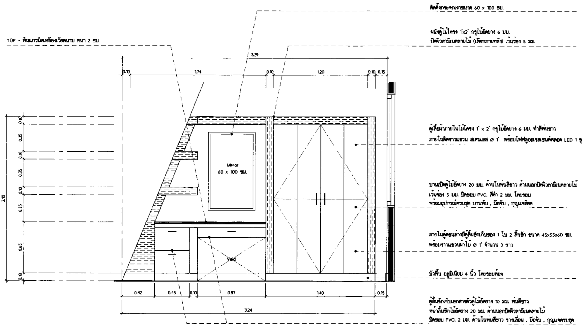
รูปตัดด้านหน้าครุภัณฑ์ (B-03) มาตราส่วน 1 : 25
